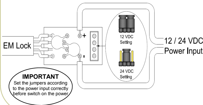
EM Lock Energized
